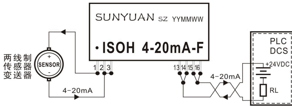
4-20mA电流环路10KV高隔离配电器IC典型应用图
