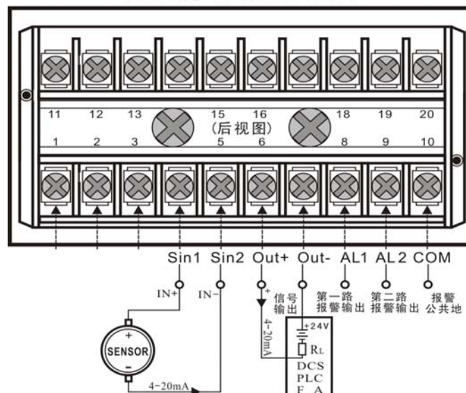
应用2:两线无源4-20mA回路馈电控制智能表 PIM-ISO 4-20mA-F-LED7
